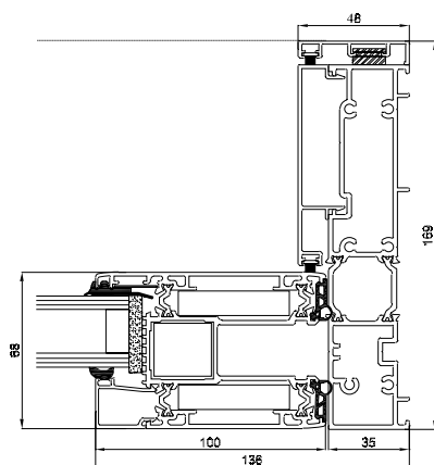
Particolare soglia ribassata - Threshold detail - Détail, seuil descendant - Türschwelle Detail
